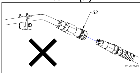
CONEXIÓN NO RECOMENDADA Desconexiones rápidas que no son de NPK (32)
